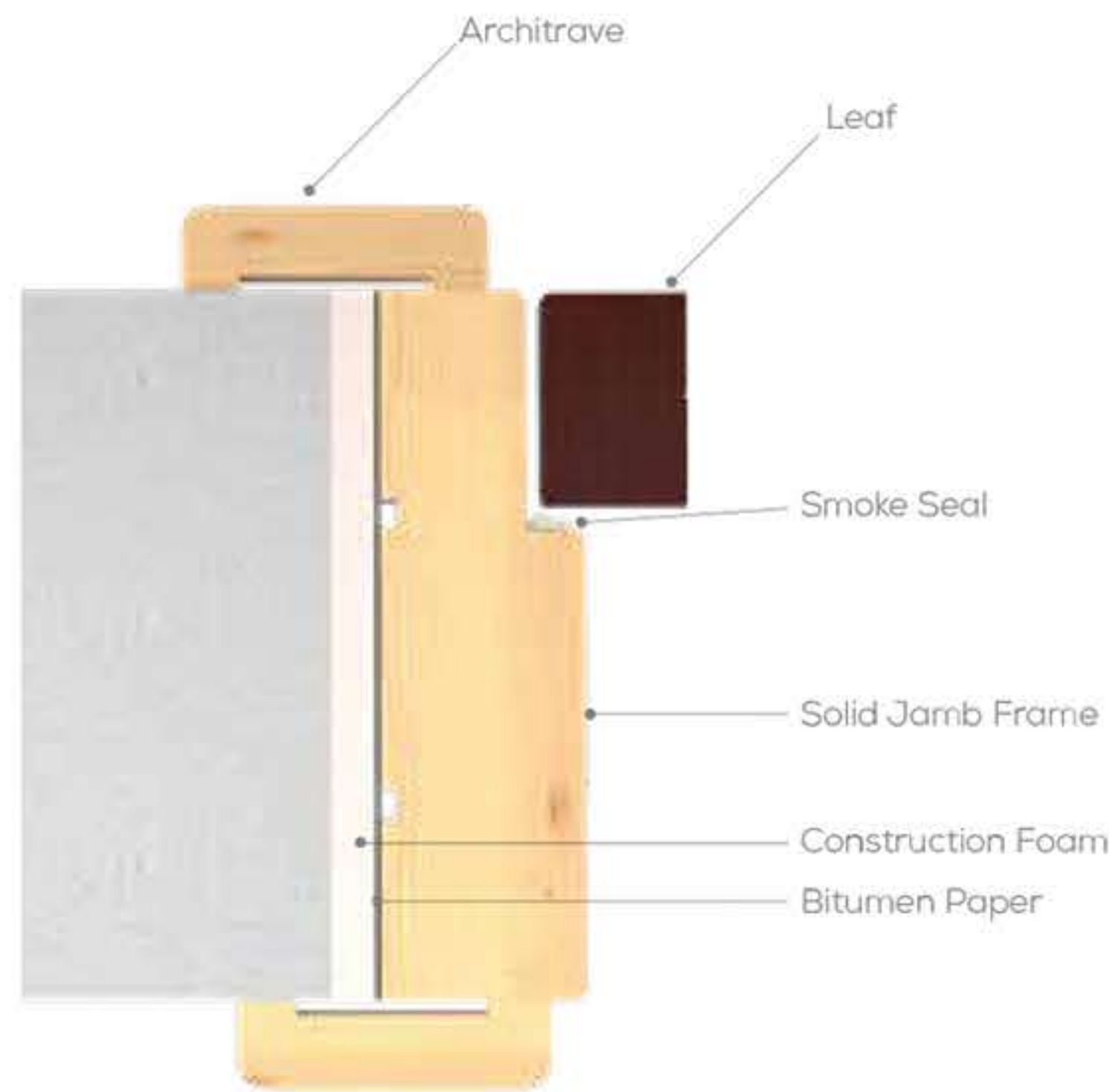
SOLID JAMB FRAME
