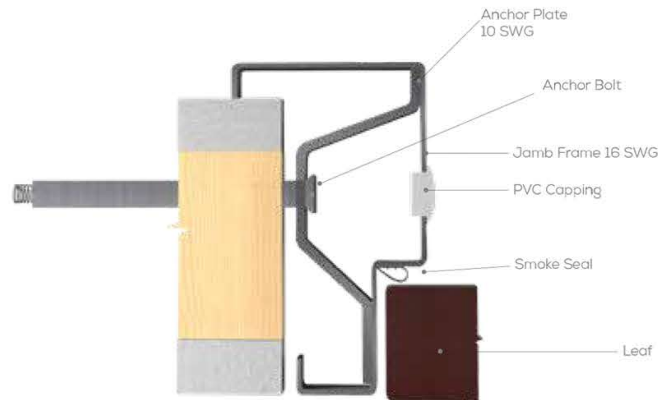
METAL JAMB FRAME
