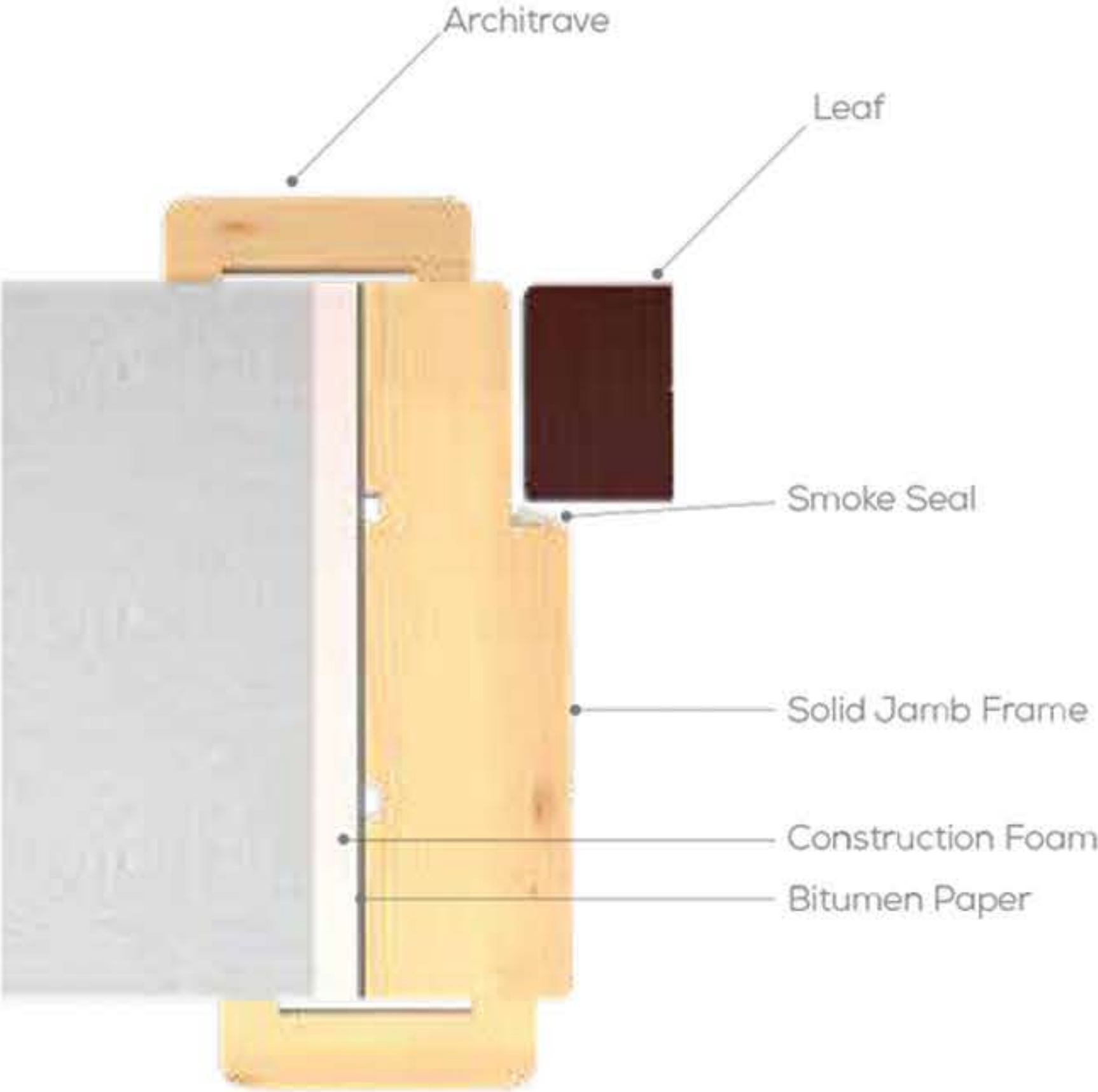
SOLID JAMB FRAME
